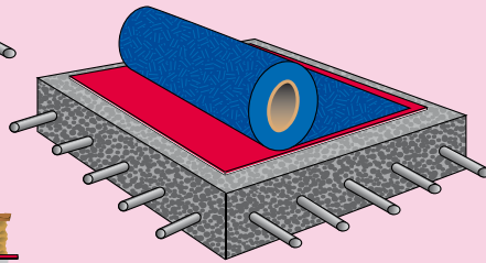
Estrich 65 mm => -55 dB
