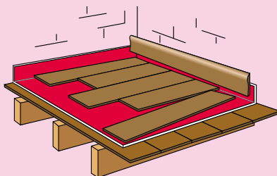
Houten vloer => -20 dB
